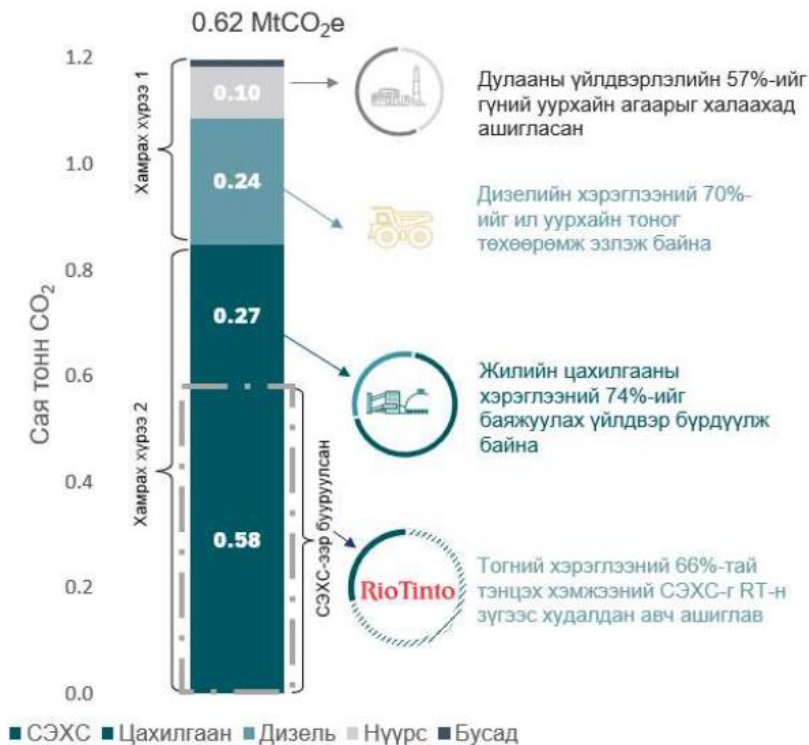
Зураг 11. 2024 оны хүлэмжийн хийн 1, 2-р хүрээний ялгарал
