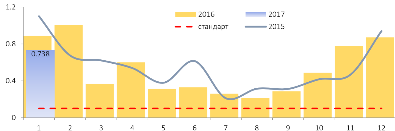
Зураг 27. Тоосны \text{PM}_{10} агууламж, \text{мг/м}^3
