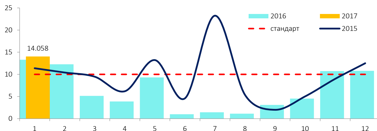
Зураг 26. Нүүрстөрөгчийн дутуу исэл, \text{мг/м}^3
